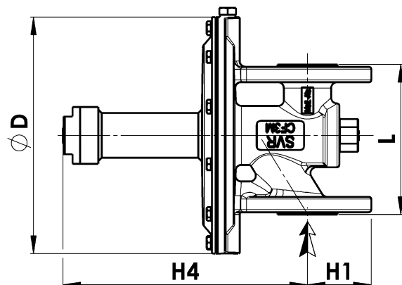
Déverseur piloté droit
