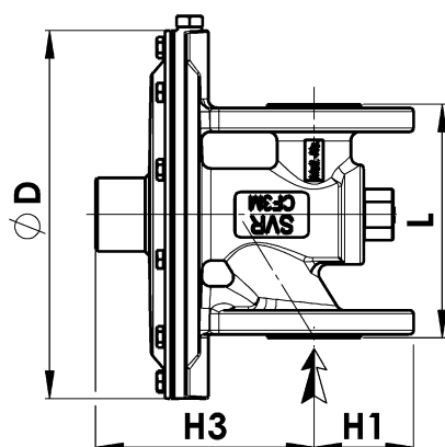
Déverseur piloté droit
