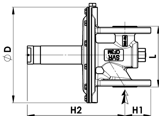
Déverseur cousin d'air droit
