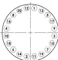
20 BOULONS 20 BOLTS
